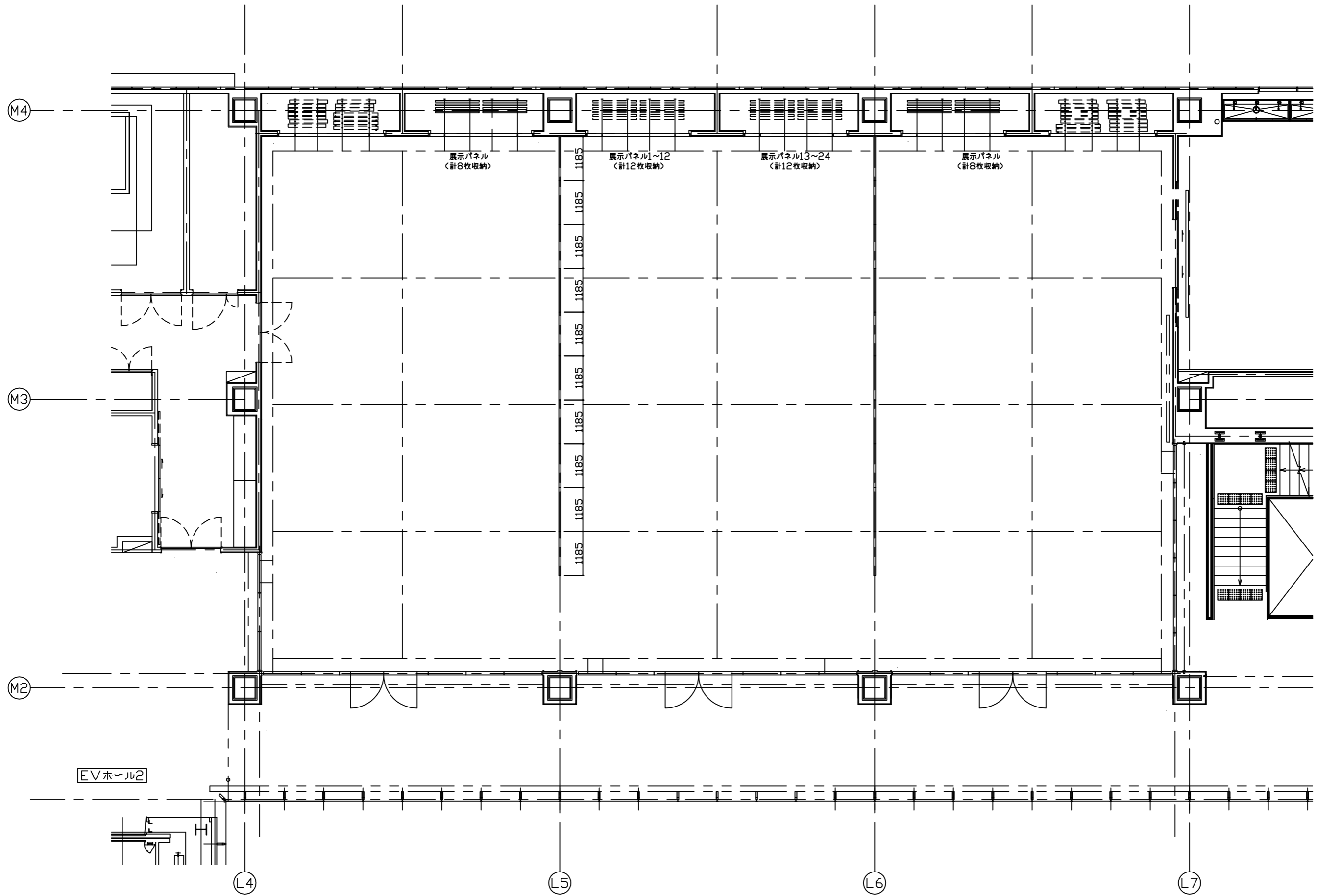
レイアウトパターン2
