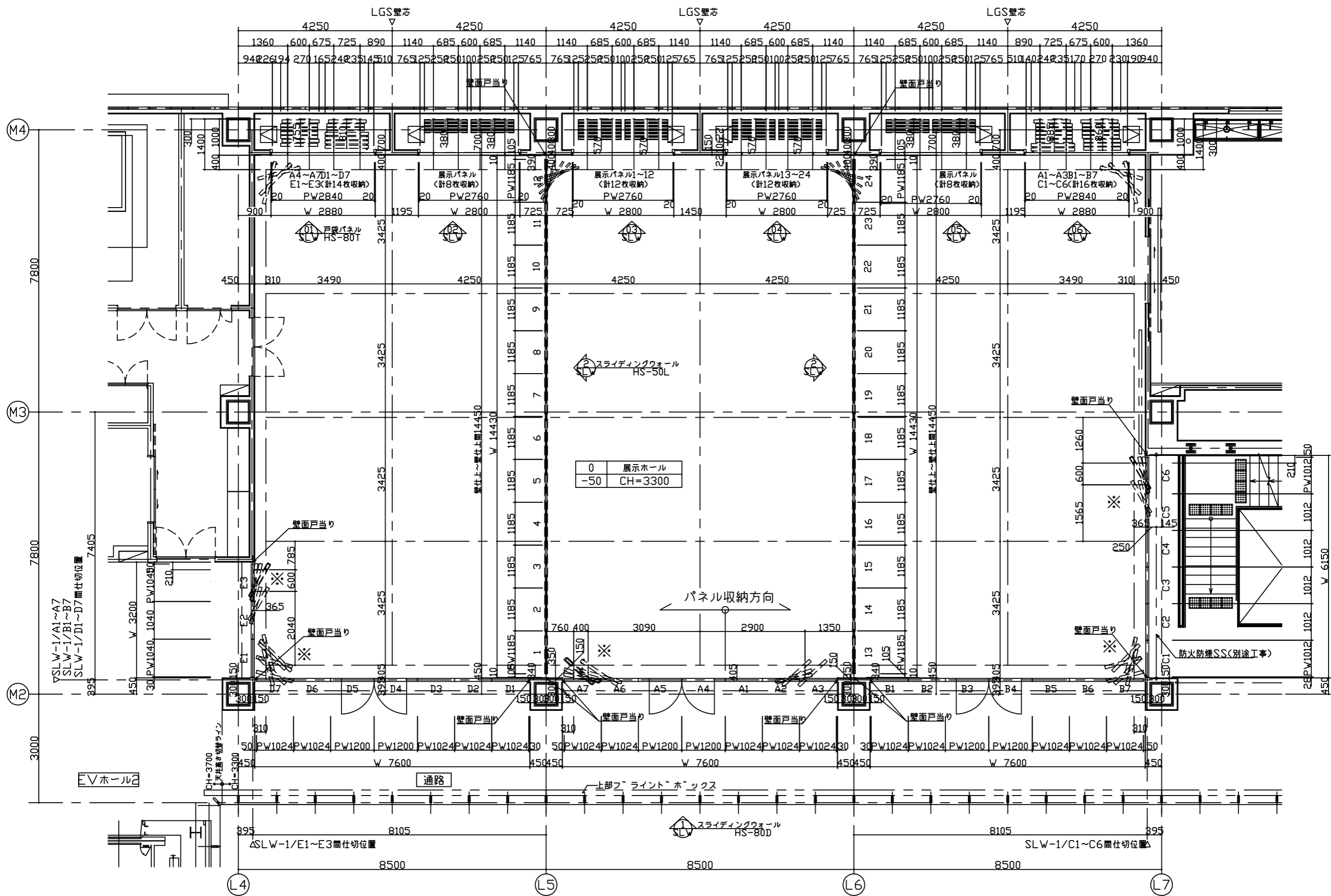
2階 展示ホール 平面図 S=1:50
