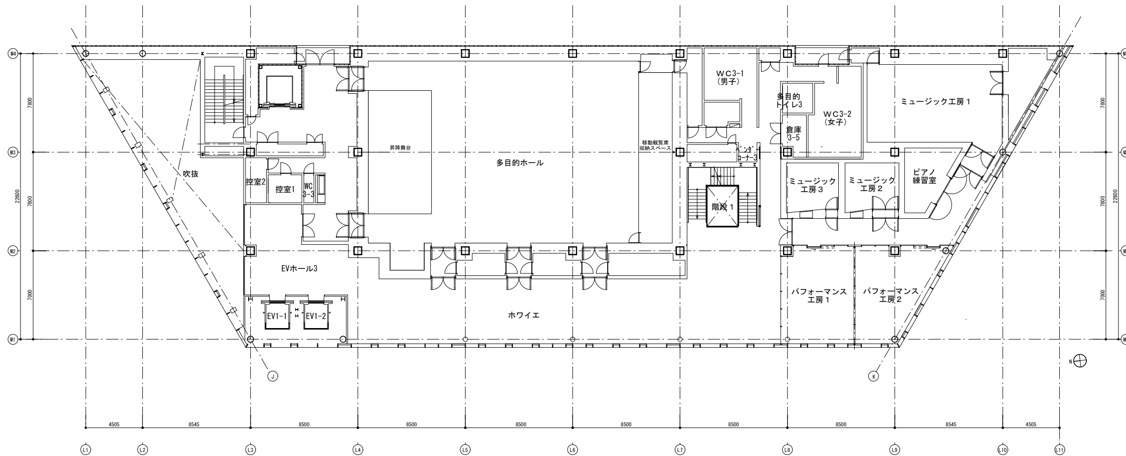
3階平面図
